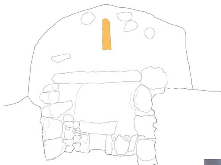
FIG. 37 – Alçado do forno de telha n.º 3 da Lagoa da Praia da Graciosa.
